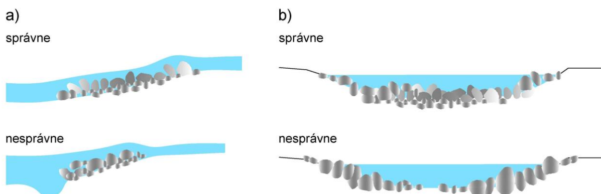
Obr. 10.10 Dnový pás z kameniva ako základný konštrukčný prvok stabilizácie prírody blízkych koryt. a) hore správne vyhotovenie dnového pásu – pás je dostatočne dlhý, dolný okraj siaha až pod dolnú relatívne upokojenú hladinu a nenastáva výraznejší prepad vody (za spoľahlivo bezpečný z hľadiska migračnej priestupnosti možno pokladať sklon pretekaného líca pásu 1 : 40), dole nesprávne vyhotovenie pásu, ktorý je krátky a na jeho dolnom okraji vzniká prepad vody, ktorý bude vymieľať koryto a objekt destabilizovať, základné hrubé kamenivo nie je doplnené kamenivom drobnejším; b) hore správne vyhotovenie – väčšina kameniva je uložená do dna koryta, čo chráni pred nadmerným zahlbovaním, dole nesprávne vyhotovenie pásu, kde je väčšina kameniva sústredená v brehoch, zatiaľ čo stabilizácia dna je nedotatočná.
