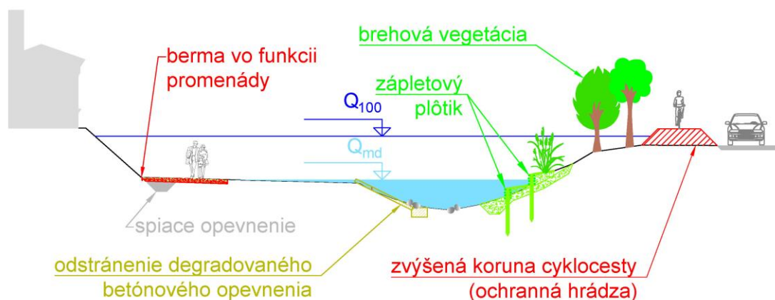
Obr.10.6 odstránenie dnového opevnenia a návrh prírody blízkeho dna
