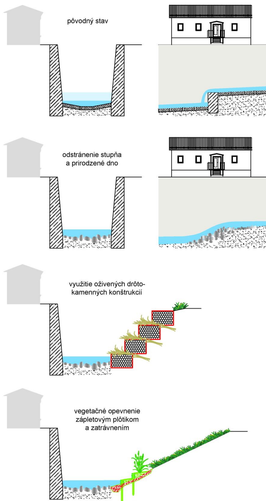
Obr.10.8 Rôzne možnosti revitalizácie tvrdo upraveného koryta
