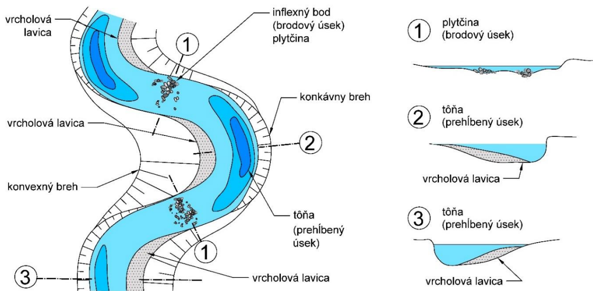
Obr.10.2 Schéma trasy zvlneného koryta – striedanie úsekov brod/tôňa
