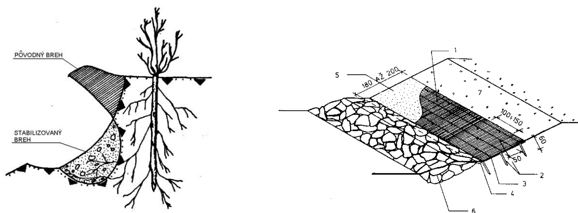
Obr. 10.12 Stabilizácia svahu palisádami (a) a rohožami z vrbového prútia (b) 1 - vrbová rohož, 2- kolíky \varnothing 6 cm, 3- spleťací drôt, 4 - zaťaženie rohože pod pätkou, 5-prekrytie zeminou, 6-päta z kamennej nahádzky, 7- ohumusovanie, osiatie (podľa Macura, Halaj, 2013)
