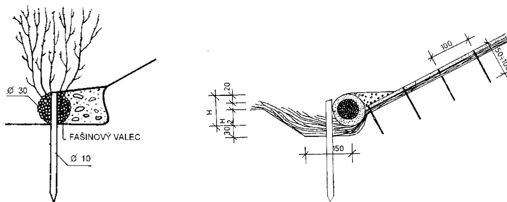
Obr. 10.15 Fašínový valec (a) (Novák a kol., 1986) a prútoštrkový ponorný valec (b) (Raplík a kol., 1989)
