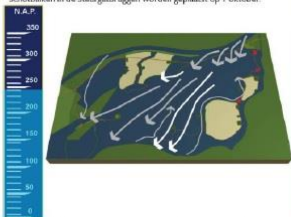
240cm +NAP: drie hoog bekade landbouwpolders stromen onder water (1/100).
