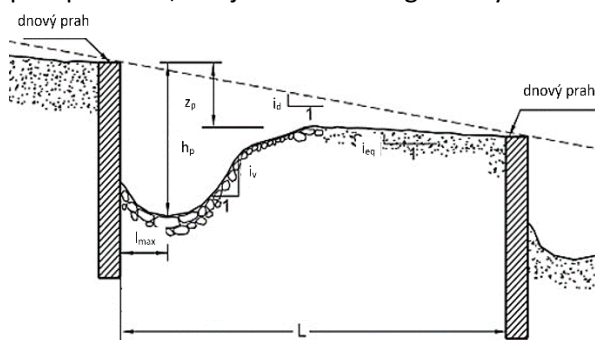
Obr. 11.7 Prevencia zanášania vodných nádrží – protierózne opatrenia v povodí nad vodnou nádržou
