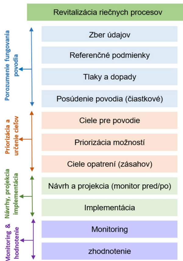
Obr.9.1 Diagram procesu revitalizácii tokov: od Analýzy povodia a pochopenie fungovania, cez stanovenie priorit (priorizácia) a cieľov, Návrhy, projekcia a realizácia, Monitorovanie a hodnotenie
