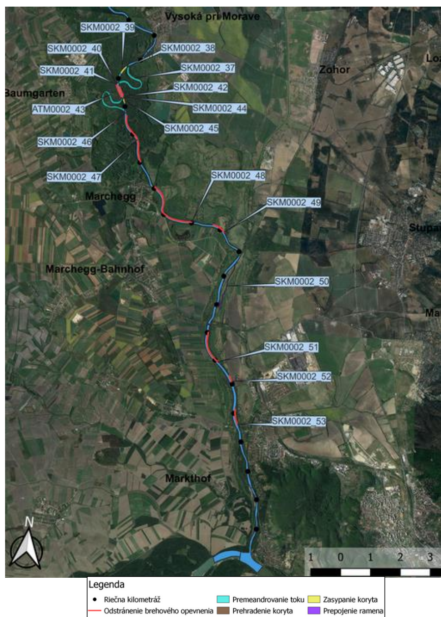
Obr. E.2 Plán opatrení na úseku Moravy medzi rkm 20-0, VÚVH 2023
