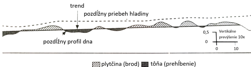
Obr. 10.3 Príklad striedania brodových a tŕňových oblastí v pozdĺžnom profile prirodzeného toku (riečka Fowey, UK, Thorne, 1997)
