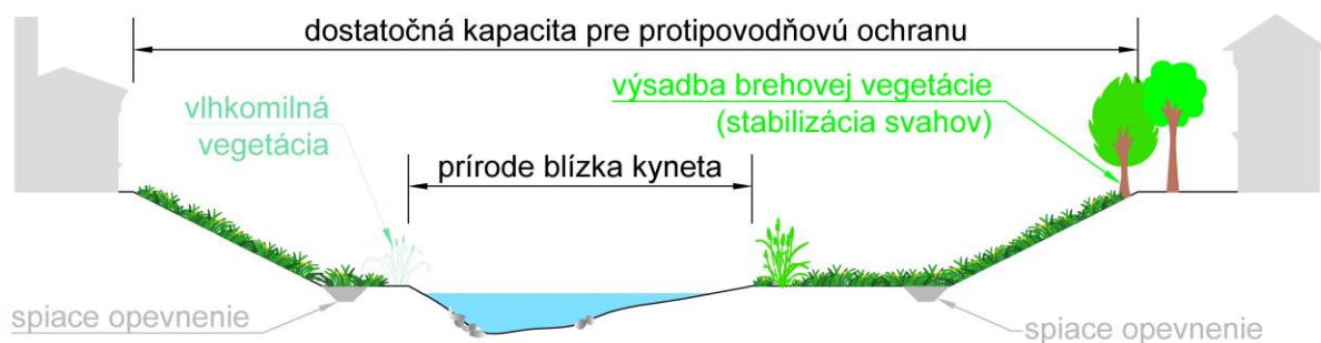
Obr. 10.5 Návrh prírody blízkej kynety v rámci starej úpravy toku
