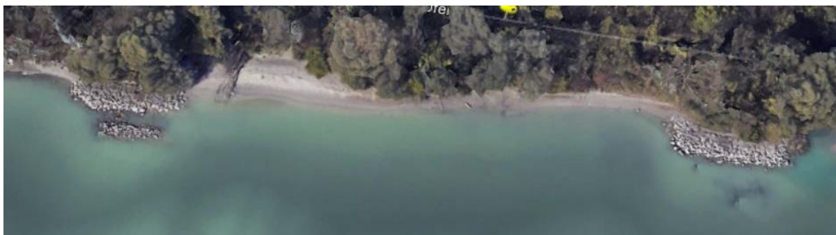
Obr. 10.7 Príklady bodového opevnenia z rieky Inn v Innsbrucku
