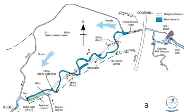
Obr.C.3 Revitalizácia rieky Cole (UK): vytvorenie nového meandrujúceho koryta menšej kapacity, ktoré zároveň umožňuje častejšie zaplavovanie inundačného územia a) schéma revitalizácie, b) pohľad na premeandrované koryto po realizácii (1996)
