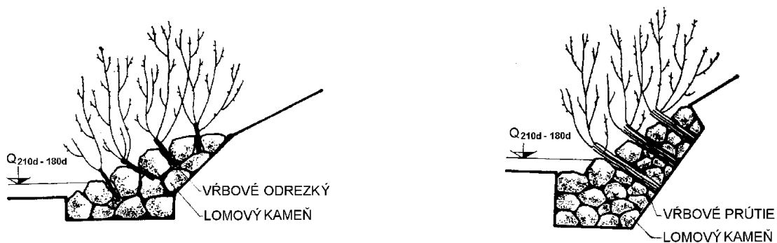
Obr. 10.16 Oživená nahádzka (a) a oživená rovnanina (b) (Novák a kol., 1986)
