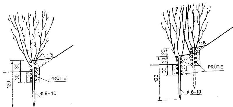
Obr. 10.13 Jednoradový a dvojradowý zápleťový plôtik (Novák a kol., 1986)
