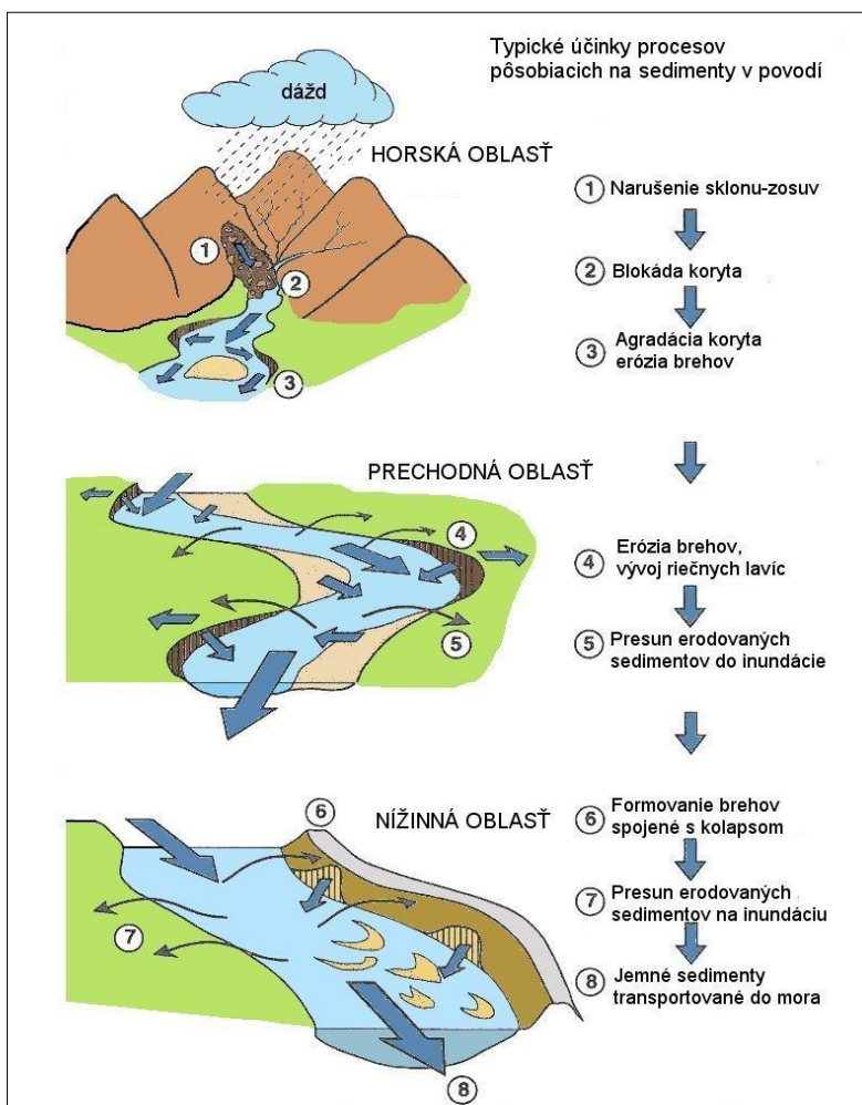
Obr.5.4 Typické účinky procesov pôsobiach na sedimenty v povodí riek (Shear a Newson, 1993)
