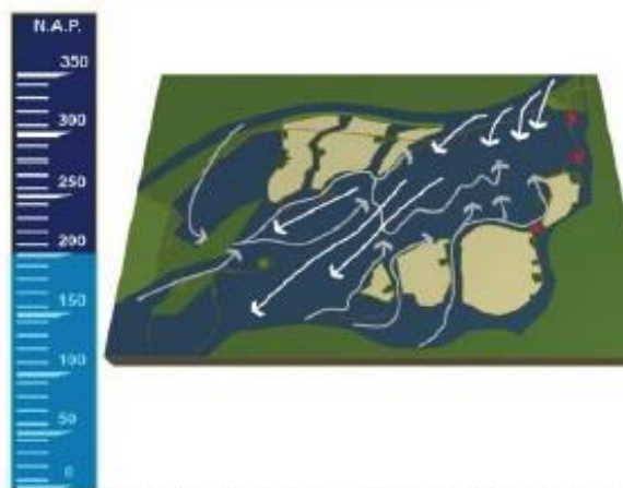
200cm +NAP: instroomdrempel stroomt over, de hoofdstroomrichting verandert.
