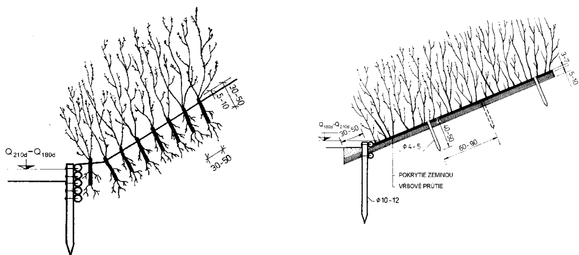
Obr. 10.11 Opevnenie svahu koryta vrbovými odrezkami (a) a prúteným obkladom (b) (podľa Novák a kol., 1986)
