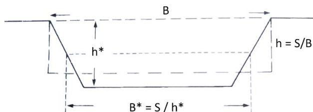
Obr.10.1 Definovanie šírky a hĺbky ktoré sa používajú v režimových rovniciach ( S =plocha priečneho profilu)
