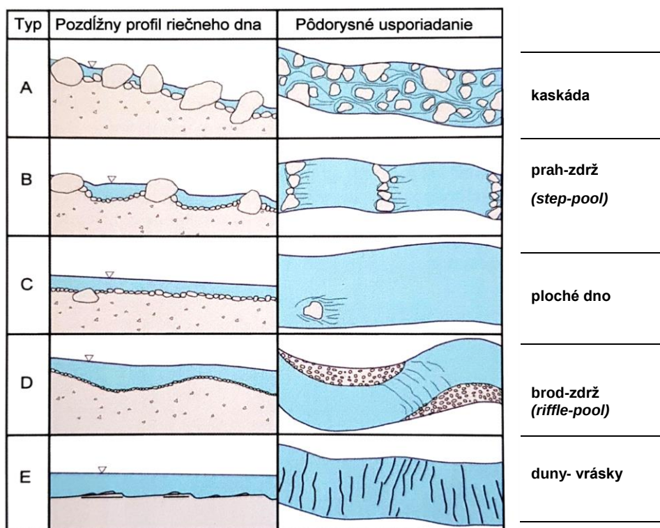
Obr.5.8 Druhá klasifikácia horských tokov podľa Montgomery & Buffington (1997)
