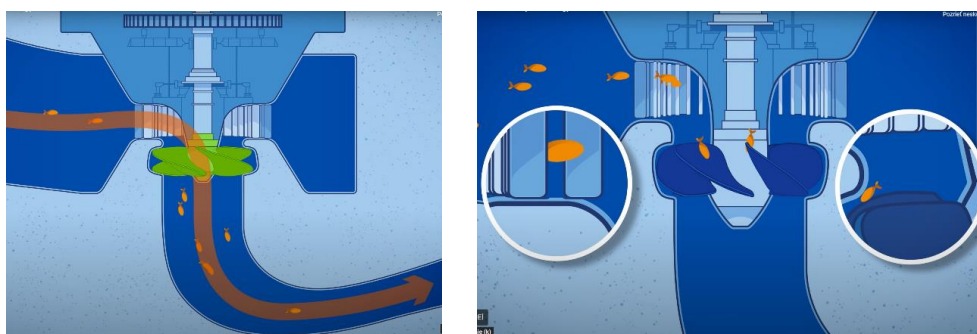
Obr. 11.9 Schéma technológie pre ryby priateľskej (fish friendly) turbíny
