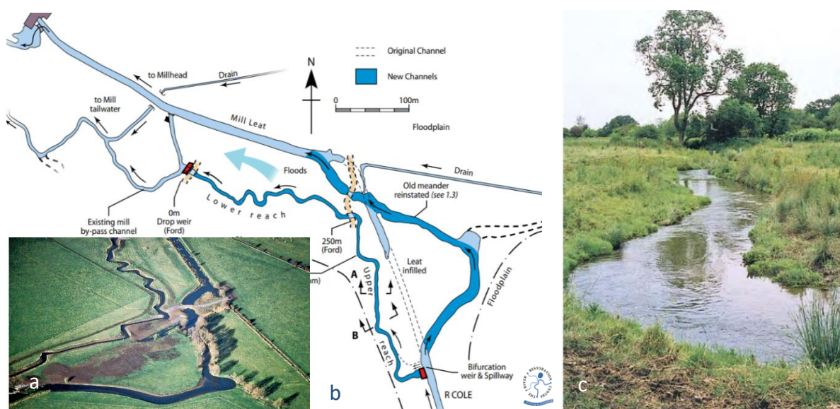
Obr.C.1 Schéma revitalizácie rieky Cole (UK) vytvorením nového meandrujúceho koryta a oživením odrezaného meandra v oblasti mlynského náhonu (River Centre), a) novovytvorené koryto rieky Cole
