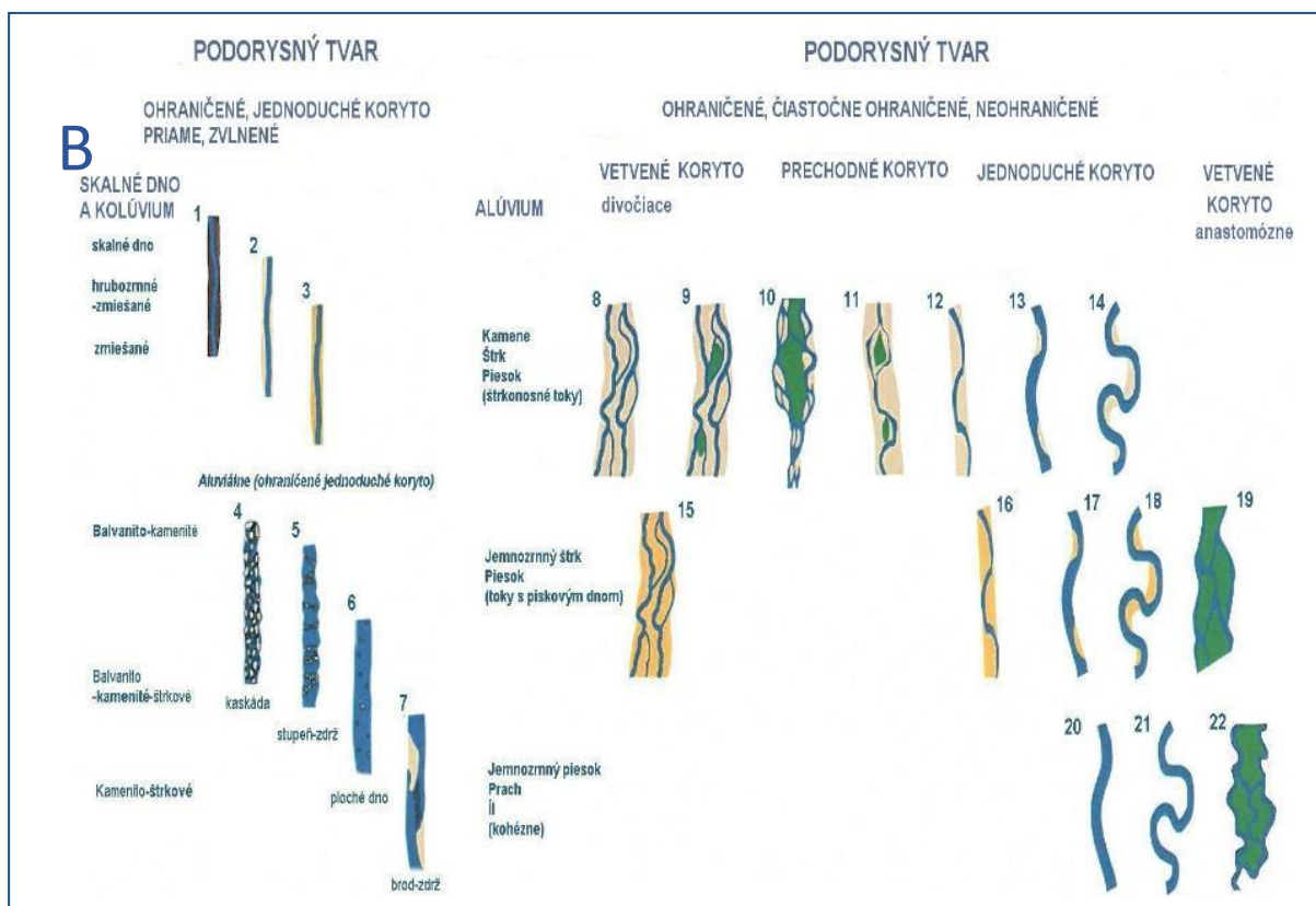
Obr.5.9 Morfológické typológia prirodzených riek – A) sedem základných typov, B) rozšírená typológia (22 typov) podľa Rinaldi et al. (REFORM, 2015)
